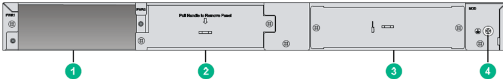
図2 背面パネル
