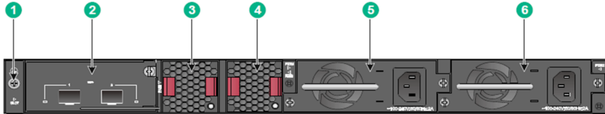
図2-5 背面パネル
