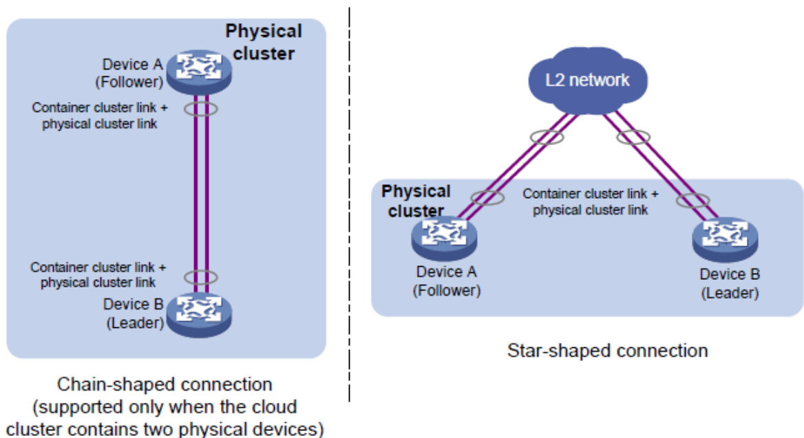
図20 物理的な接続トポロジ
