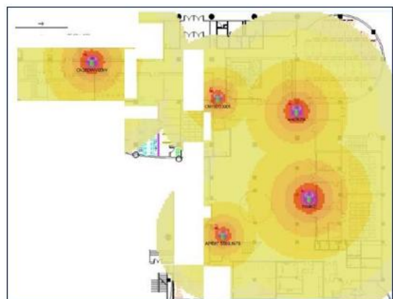
図 WSM信号強度のシュミレーション 図 WSM信号強度の表示
