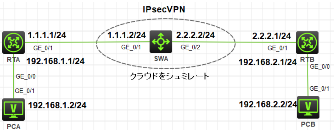
図 4.1 実習ネットワーク
