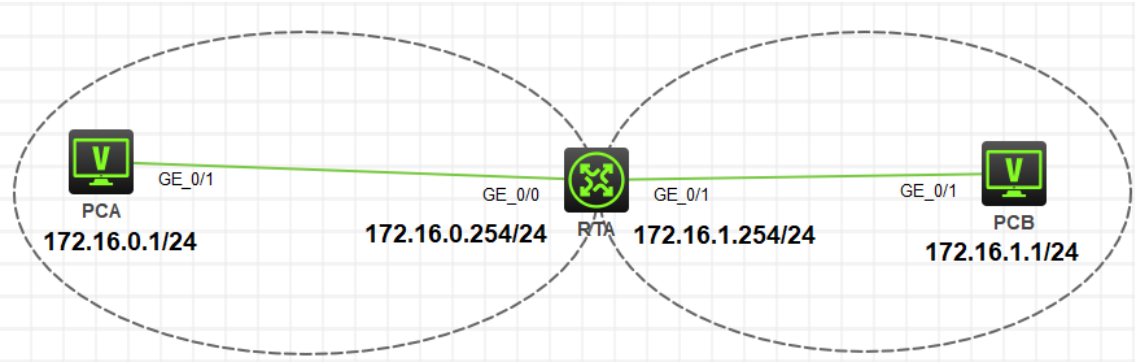
図 7.1 実習ネットワーク
