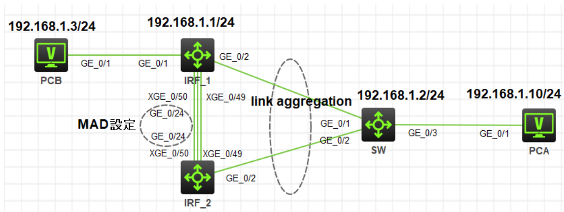
図 1.5 実習ネットワーク
