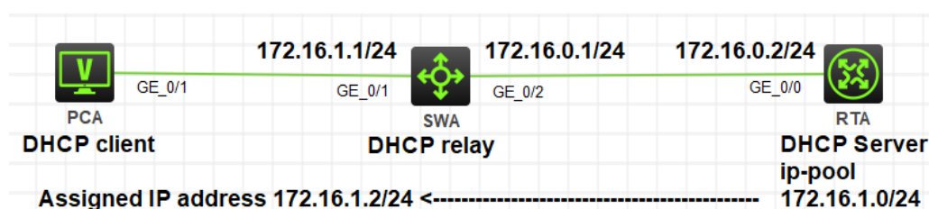
図 8.5 実習ネットワーク
