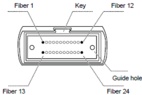
図6 24ファイバーコネクタの端面
